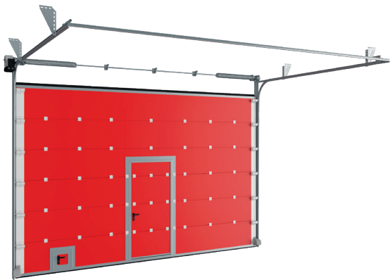
■ Секционные противопожарные ворота с пределом огнестойкости EI 60
